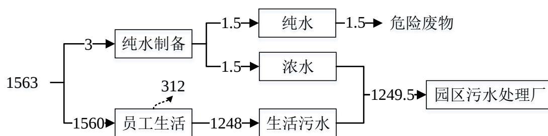
图 2-1 水平衡图
