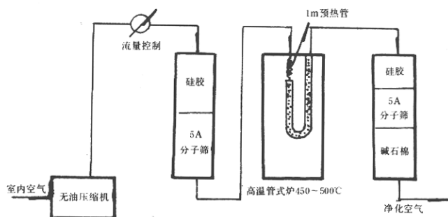
图 A1 除烃净化空气装置
